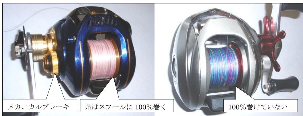
図 4 6、糸の巻き方
